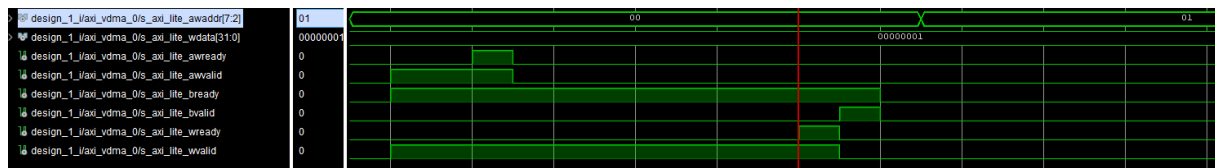
FIGURE 14 : ANALYSE SUR L'ILA DES SIGNAUX DE VDMA
